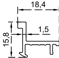
كلبس قصير زجاج (13-18) ملم الرقم التسلسلي للصنف: BLT3164 الوزن 0.157: (Kg/m)
