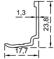
كلبس عالي زجاج 2.4 ملم الرقم التسلسلي للصنف: BLT3419 الوزن 0.141: (Kg/m)
