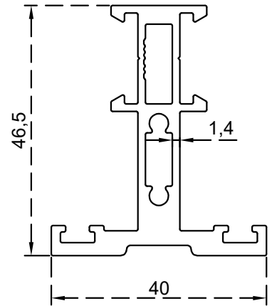
BLT775: الرقم التسلسلي للصنف: الوزن 0.991:(Kg/m)
