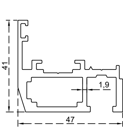
دفة زجاج عادي مع كسحة الرقم التسلسلي للصنف: BLT1980 الوزن 1.123:(Kg/m)
