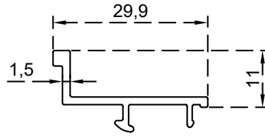
كلبس قصير زجاج (3-6) ملم الرقم التسلسلي للصنف: BLT766 الوزن 0.205: (Kg/m)
