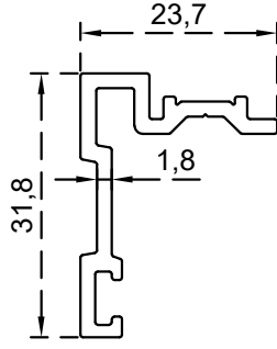
BLT771: الرقم التسلسلي للصنف: الوزن 0.363:(Kg/m)
