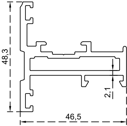
دفة فتحة خارجية 48.3 ملم الرقم التسلسلي للصنف: BLT758 الوزن 1.119:(Kg/m)
