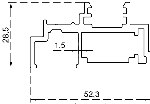
دفة وسط زجاج دبل الرقم التسلسلي للصنف: BLT1970 الوزن 0.976:(Kg/m)
