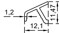
اف مايم 12.10 ملم الرقم التسلسلي للصنف: BLT3898 الوزن 0.097:(Kg/m)
