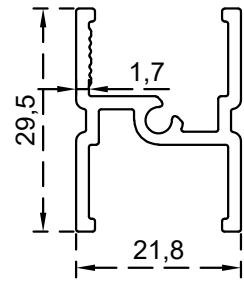
BLT747: الرقم التسلسلي للصنف: الوزن 0.417:(Kg/m)
