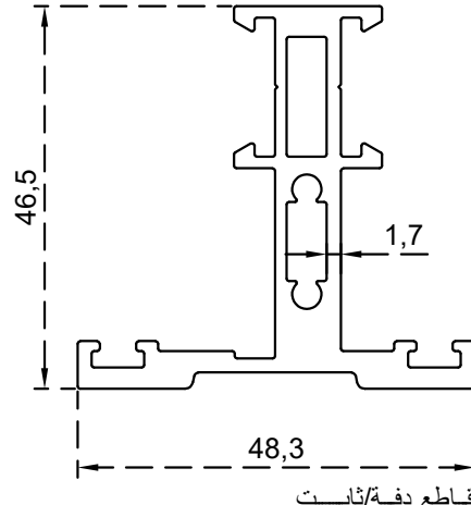
قاطع دفة/ثابت الرقم التسلسلي للصنف: BLT773 الوزن 1.094:(Kg/m)
