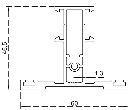
قاطع دفة/دفة الرقم التسلسلي للصنف: BLT761 الوزن 0.990:(Kg/m)
