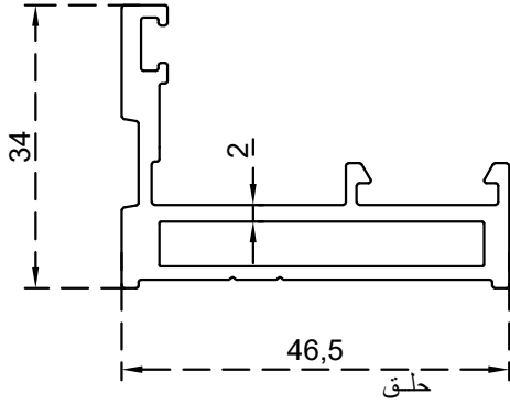
BLT3188: الرقم التسلسلي للصنف: الوزن 0.823:(Kg/m)
