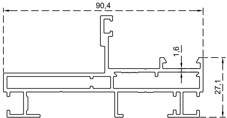
ثابت مجريين 90 ملم الرقم التسلسلي للصنف: BLT3791 الوزن 1.411:(Kg/m)
