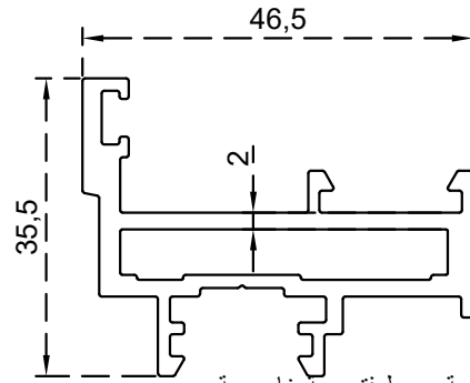
دفة وسط فتحة خارجية الرقم التسلسلي للصنف: BLT3187 الوزن (Kg/m): 0.910
