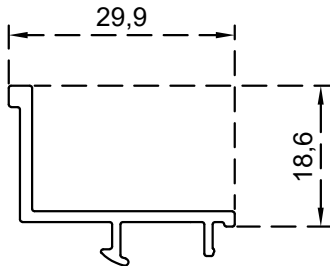
كابس عالي زجاج (6-3) ملم الرقم التسلسلي للصنف: BLT1979 الوزن 0.231:(Kg/m)
