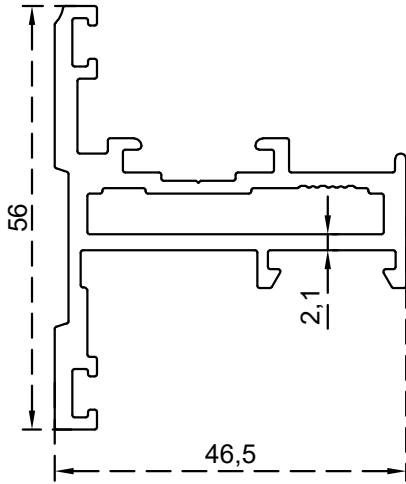
دفة فتحة خارجية 56 ملم الرقم التسلسلي للصنف: BLT4952 الوزن (Kg/m): 1.151
