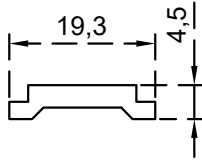
فلاخ الرقم التسلسلي للصنف: BLT1756 الوزن 0.157: (Kg/m)
