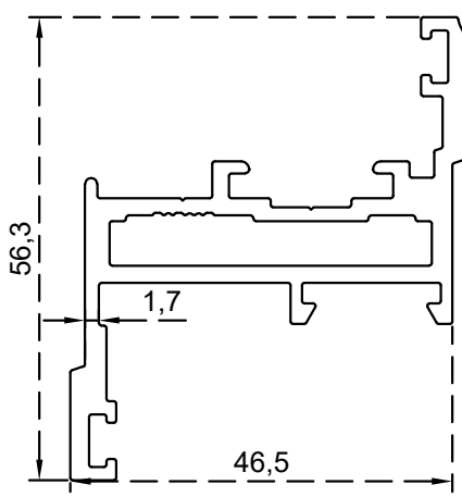
BLT757: الرقم التسلسلي للصنف: الوزن 1.144:(Kg/m)
