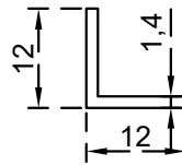
زاوية حلق الرقم التسلسلي للصنف: J12X12X1.4 الوزن 0.085: (Kg/m)
