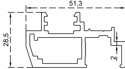
دفة وسط زجاج دبل مع كسحة الرقم التسلسلي للصنف: BLT4400 الوزن (Kg/m): 0.952
