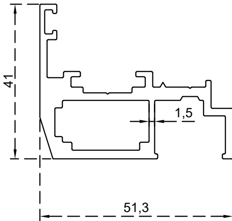
دفة زجاج دبل مع كسحة الرقم التسلسلي للصنف: BLT1981 الوزن 1.117:(Kg/m)
