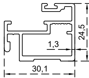
منخل متحرك الرقم التسلسلي للصنف: BLT4290 الوزن 0.484:(Kg/m)
