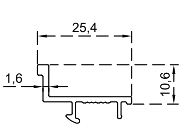
كلبس قصير زجاج (6-11) ملم الرقم التسلسلي للصنف: BLT3601 الوزن 0.180: (Kg/m)
