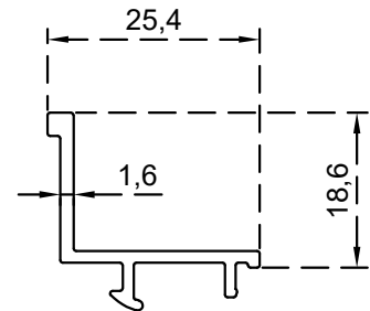
كابس عالي زجاج (11-6) ملم الرقم التسلسلي للصنف: BLT1901 الوزن 0.281:(Kg/m)
