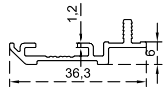
برواز بلجي الرقم التسلسلي للصنف: BLT760 الوزن 0.235: (Kg/m)
