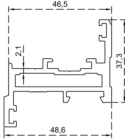
دفة باب فتحة داخلية الرقم التسلسلي للصنف: BLT759 الوزن 1.168:(Kg/m)
