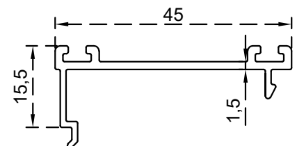
غطاء تحتون باب مع فرش ايتين ZD007: الرقم التسلسلي للصنف: الوزن 0.318:(Kg/m)
