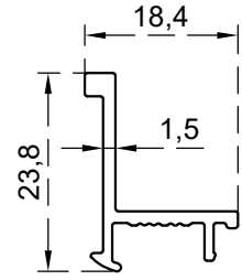
كلبس قصير زجاج (13-18) ملم الرقم التسلسلي للصنف: BLT3163 الوزن 0.190: (Kg/m)
