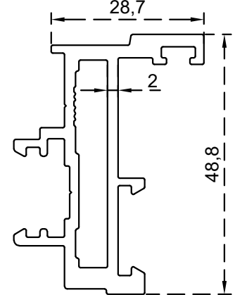
دفة وسط فتحة داخلية الرقم التسلسلي للصنف: BLT772 الوزن 0.998:(Kg/m)
