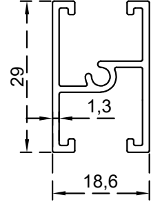
قاطع دفة زجاج عادي الرقم التسلسلي للصنف: BLT1572 الوزن 0.351:(Kg/m)
