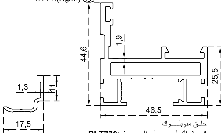
BLT770: الرقم التسلسلي للصنف: الوزن 1.020:(Kg/m)
