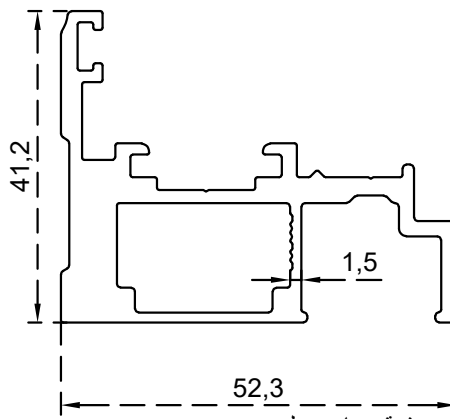
دفة زجاج دبل الرقم التسلسلي للصنف: BLT776 الوزن 1.216:(Kg/m)
