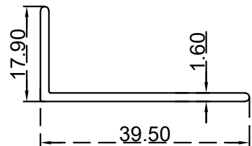
زاوية (39.5X17.9X1.6) ملم الرقم التسلسلي للصف: J39.5X17.9X1.6 (الوزن (Kg/m): 0.241)
