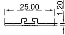
قاعدة فرشاية الرقم التسلسلي للصنف: BLT3631 (الوزن 0.104: (Kg/m
