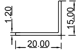
زاوية (20X15X1.2) ملم الرقم التسلسلي للصف: BLT3541 (الوزن (Kg/m): 0.110)
