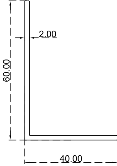
زاوية (0.9*15*20) ملم الرقم التسلسلي للصنف: J60X40X2 الوزن 0.533:(Kg/m)
