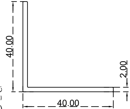
زاوية (40X40X2) ملم الرقم التسلسلي للصف: BLT3610 (الوزن 0.424: (Kg/m)
