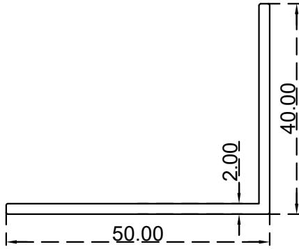
زاوية (50X40X2) ملم الرقم التسلسلي للصنف: J50X40X2 (الوزن 0.478: (Kg/m
