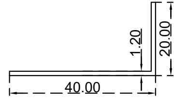
زاوية (40X20X1.2) ملم الرقم التسلسلي للصف: J40X20X1.2 (الوزن 0.194: (Kg/m)
