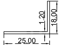
زاوية (25X18X1.2) ملم الرقم التسلسلي للصف: J25X18X1.2 (الوزن (Kg/m): 0.136)
