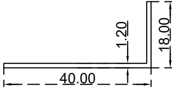
زاوية (40X18X1.2) ملم الرقم التسلسلي للصف: J40X18X1.2 (الوزن 0.185: (Kg/m)
