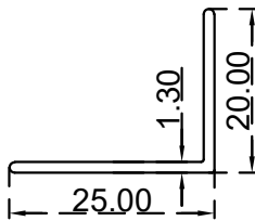
زاوية (25X20X1.3) ملم الرقم التسلسلي للصف: J25X20X1.3 (الوزن (Kg/m): 0.154)
