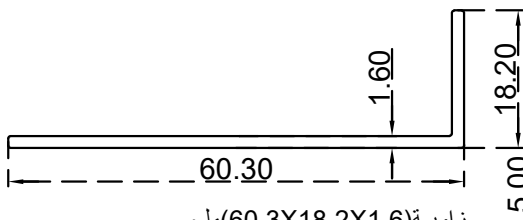
زاوية (60.3X18.2X1.6) ملم الرقم التسلسلي للصنف: J60.3X18.2X1.6 (الوزن 0.334: (Kg/m
