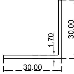
زاوية (30X30X1.7) ملم الرقم التسلسلي للصف: J30X30X1.7 (الوزن 0.269: (Kg/m)
