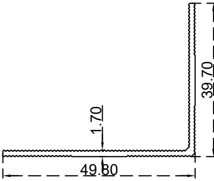
زاوية (49.8X39.7X1.7) ملم الرقم التسلسلي للصف: BLT972 (الوزن 0.346: (Kg/m)
