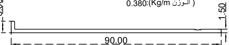
زاوية (90X5X1.5) ملم الرقم التسلسلي للصنف: BLT3486 (الوزن 0.380: (Kg/m
