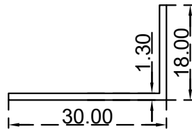
زاوية (30X18X1.3) ملم الرقم التسلسلي للصف: J30X18X1.3 (الوزن (Kg/m): 0.164)
