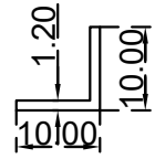
زاوية (10X10X1.2) ملم الرقم التسلسلي للصف: J10X10X1.2 (الوزن (Kg/m): 0.062)
