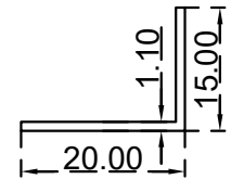
زاوية (20X15X1.1) ملم الرقم التسلسلي للصف: J20X15X1.1 (الوزن (Kg/m): 0.101)
