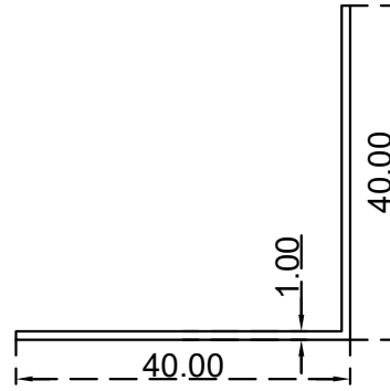
زاوية (40X40X1) ملم الرقم التسلسلي للصف: J40X40X1 (الوزن 0.214: (Kg/m)
