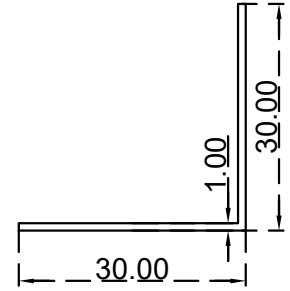
زاوية (30X30X1) ملم الرقم التسلسلي للصف: J30X30X1A (الوزن 0.160: (Kg/m)
