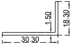
زاوية (30.3X18.3X1.5) ملم الرقم التسلسلي للصف: J30.3X18.3X1.5 (الوزن (Kg/m): 0.192)
