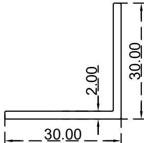
زاوية (30X30X2) ملم الرقم التسلسلي للصف: J30X30X2H (الوزن (Kg/m): 0.315)
