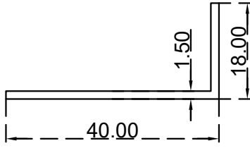
زاوية (40X18X1.5) ملم الرقم التسلسلي للصف: J40X18X1.5 (الوزن 0.230: (Kg/m)
