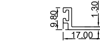
زاوية مع فرشاية (17X9.8X1.3) ملم الرقم التسلسلي للصنف: BLT1576 (الوزن 0.104: (Kg/m
