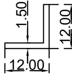
زاوية (12X12X1.5) ملم الرقم التسلسلي للصف: J12X12X1.5 (الوزن (Kg/m): 0.089)
