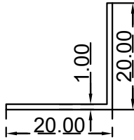
زاوية (20X20X1) ملم الرقم التسلسلي للصف: J20X20X1 (الوزن (Kg/m): 0.106)
