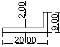
زاوية (20X9X2) ملم الرقم التسلسلي للصف: CPT16 (الوزن (Kg/m): 0.146)
