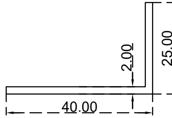
زاوية (40X25X2) ملم الرقم التسلسلي للصف: J40X25X2 (الوزن 0.343: (Kg/m)
