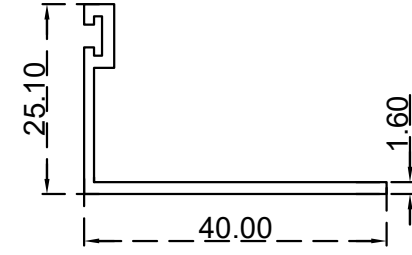
زاوية مع فرشاية (40X25.1X1.6) ملم الرقم التسلسلي للصف: BLT061 (الوزن (Kg/m): 0.293)
