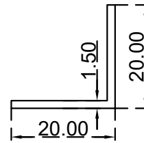
زاوية (20X20X1.5) ملم الرقم التسلسلي للصف: J20X20X1.5 (الوزن (Kg/m): 0.157)
