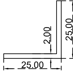
زاوية (25X25X2) ملم الرقم التسلسلي للصف: J25X25X2B (الوزن (Kg/m): 0.261)
