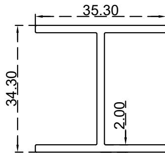
H(35.3*34.4*2)mm الرقم التسلسلي للصنف: GC35.3*34.3*2 الوزن 0.549:(Kg/m)
