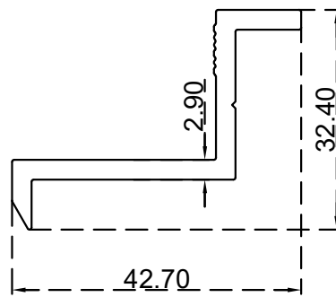
اند كلامب 44 ملم الرقم التسلسلي للصنف: BLT1998 الوزن 0.555:(Kg/m)
