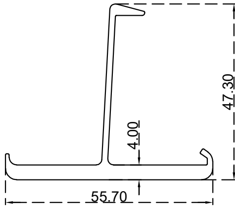
بروفيل زاوية جمع 1 الرقم التسلسلي للصنف: BLT227 الوزن 0.859:(Kg/m)
