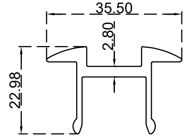
مشبك كلامب وسط الرقم التسلسلي للصنف: BLT2000 الوزن 0.455:(Kg/m)
