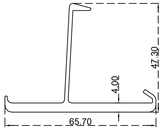
بروفيل زاوية جمع 2 الرقم التسلسلي للصنف: BLT229 الوزن 0.979:(Kg/m)
