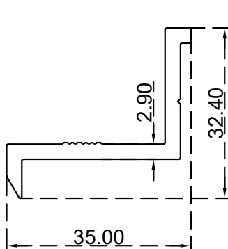
بروفيل زاوية جمع 3 الرقم التسلسلي للصنف: BLT228 الوزن 0.985:(Kg/m)
