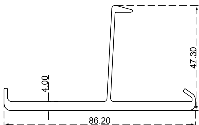
بروفيل زاوية جمع 4 الرقم التسلسلي للصنف: BLT230 الوزن 1.218:(Kg/m)
