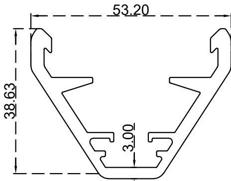
بروفيل بركس 2 الرقم التسلسلي للصنف: BLT3280 الوزن 1.143:(Kg/m)
