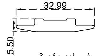
بروفيل بركس 3 الرقم التسلسلي للصنف: BLT3281 الوزن 0.331:(Kg/m)
