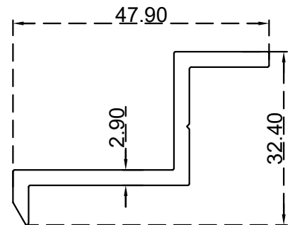
اند كلامب 55 ملم الرقم التسلسلي للصنف: BLT1999 الوزن 0.600:(Kg/m)
