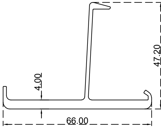
بروفيل زاوية جمع 3 الرقم التسلسلي للصنف: BLT228 الوزن 0.985:(Kg/m)
