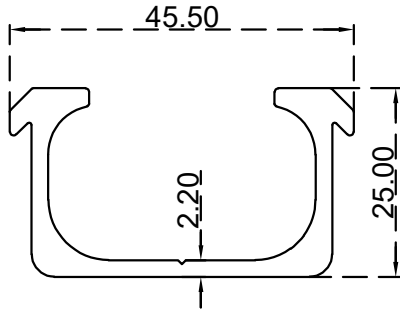
بروفيل بركس 1 الرقم التسلسلي للصنف: BLT3279 الوزن 0.750:(Kg/m)
