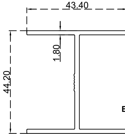
H(43.4*44*1.8)mm الرقم التسلسلي للصنف: BLT3604 الوزن 0.650:(Kg/m)
