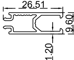
ارتفاع لزجاج 24 ملم الرقم التسلسلي للصنف: BLT4739 الوزن 0.215:(Kg/m)
