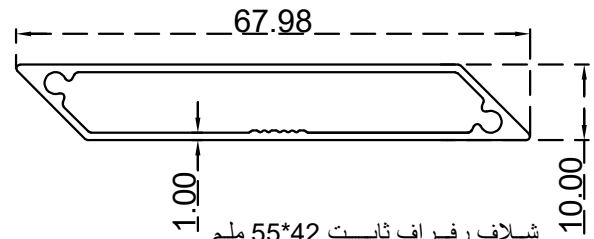
شلاف رفراف ثابت 55*42 ملم الرقم التسلسلي للصنف: BLT4731 الوزن 0.414:(Kg/m)
