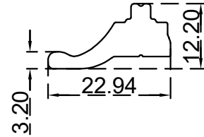
حامل زجاج 11 ملم الرقم التسلسلي للصنف: BLT4781 الوزن 0.332:(Kg/m)
