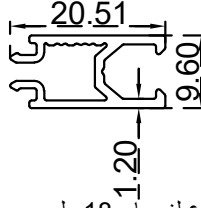
ارتفاع لزجاج 18 ملم الرقم التسلسلي للصنف: BLT4737 الوزن 0.178:(Kg/m)
