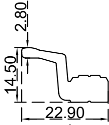
حامل زجاج 10 ملم الرقم التسلسلي للصنف: BLT4734 الوزن 0.340:(Kg/m)
