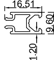
ارتفاع لزجاج 14 ملم الرقم التسلسلي للصنف: BLT4738 الوزن 0.150:(Kg/m)
