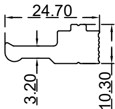
موصل زجاج عازل لاطار ثابت الرقم التسلسلي للصنف: BLT4902 الوزن 0.405:(Kg/m)
