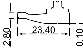
حامل زجاج 10.5 ملم الرقم التسلسلي للصنف: BLT4780 الوزن 0.331:(Kg/m)
