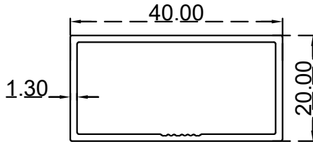
مستطيل 1.3*20*40 ملم الرقم التسلسلي للصنف: FG40X20X1.3 الوزن 0.402:(Kg/m)
