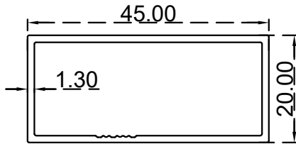
مستطيل 1.3*20*45 ملم الرقم التسلسلي للصنف: FG45X20X1.3 الوزن 0.437:(Kg/m)
