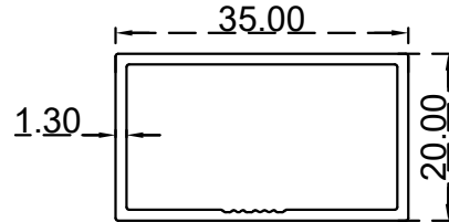
مستطيل 1.3*20*35 ملم الرقم التسلسلي للصنف: FG35X20X1.3 الوزن 0.367:(Kg/m)
