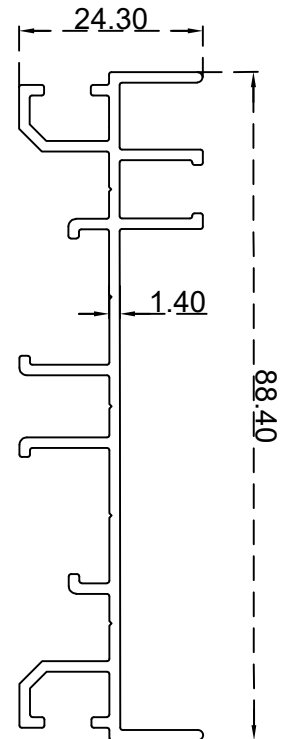
الرقم التسلسلي للصنف: BLT1571 الوزن ( Kg/m ) : 0.8220
