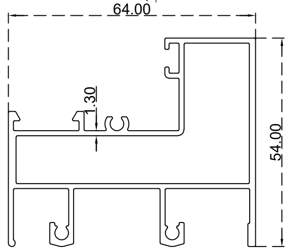
امباطية مجريين و نصف مع ثابت الرقم التسلسلي للصف: BLT1902 الوزن ( Kg/m ): 1.1860
