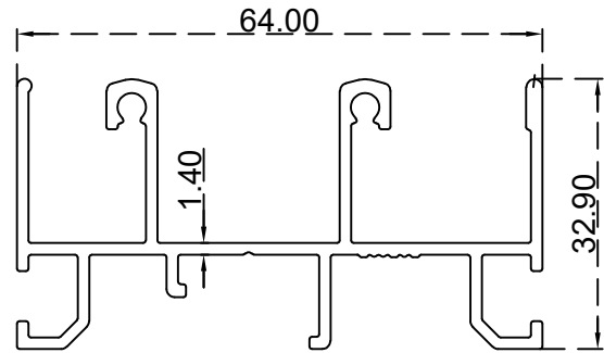
عليون مجريين و نصف الرقم التسلسلي للصف: ZD034 الوزن ( Kg/m ): 0.8750
