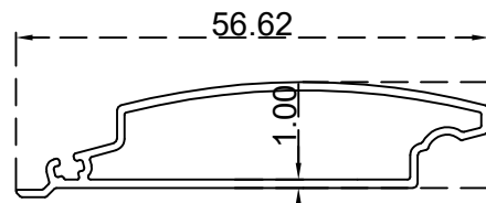
شلاف 50 ملم الرقم التسلسلي للصف: ZD009B الوزن (Kg/m): 0.328
