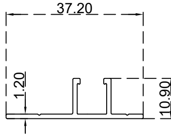
يو حلق الرقم التسلسلي للصف: BLT1590 الوزن (Kg/m): 0.19
