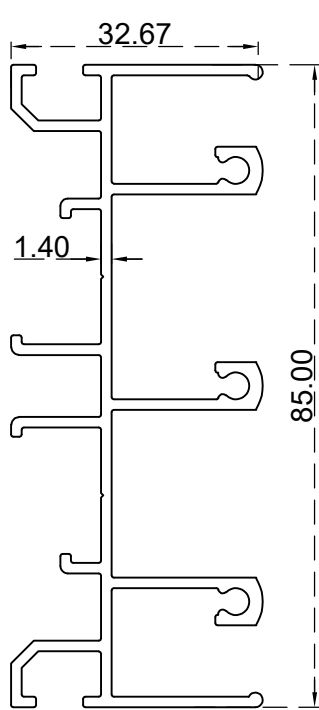
الرقم التسلسلي للصنف: BLT1566 الوزن ( Kg/m ) : 1.1530
