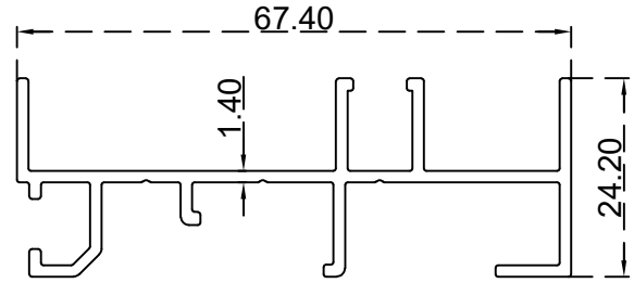
جنب مجريين و نصف عادي شمال الرقم التسلسلي للصنف: ZD032 الوزن ( Kg/m ) : 0.660
