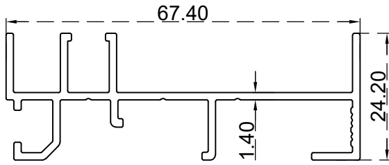
جنب مجريين و نصف عادي يمين الرقم التسلسلي للصنف: ZD033 الوزن ( Kg/m ) : 0.6630
