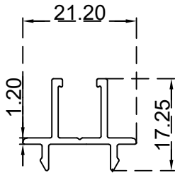
نوشيك أربع دفات الرقم التسلسلي للصف: BLT1589 الوزن (Kg/m): 0.1780
