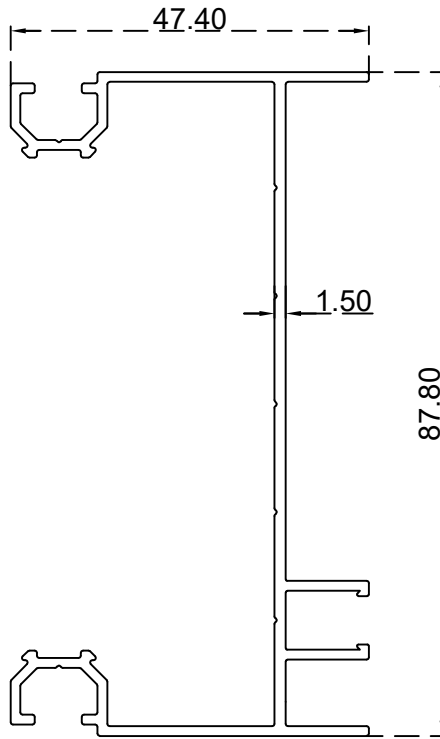
الرقم التسلسلي للصنف: BLT1571 الوزن ( Kg/m ) : 0.9090
