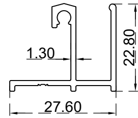
أرضية مجرى واحد 23 ملم الرقم التسلسلي للصف: BLT3521 الوزن (Kg/m): 0.2930
