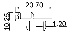
قاعدة بي كيس الرقم التسلسلي للصف: BLT1939 الوزن ( Kg/m ): 0.128
