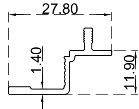
زد منخل الرقم التسلسلي للصف: BLT3620 الوزن (Kg/m): 0.1870
