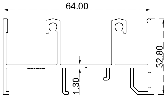
عليون مجريين ونصف مع فرزة برواز الرقم التسلسلي للصنف: BLT3149 الوزن ( Kg/m ) : 0.7930
