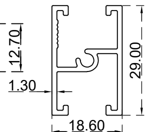
قاطع عادي (6-3) ملم الرقم التسلسلي للصف: BLT1572 الوزن (Kg/m): 0.3510
