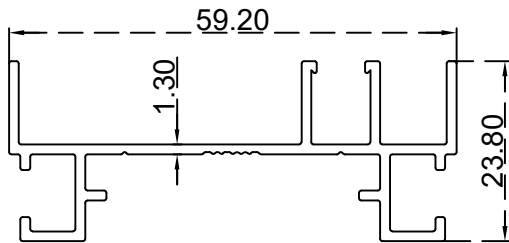
جنب مجريين عادي مع فرزتين برواز الرقم التسلسلي للصنف: BLT3637 الوزن ( Kg/m ) : 0.5470
