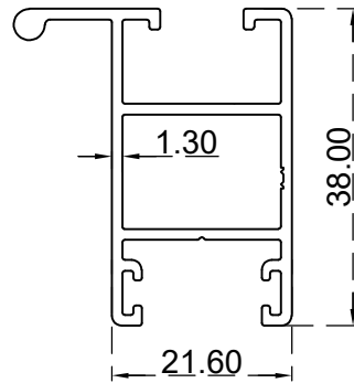
سادة مقوى (6-3) ملم الرقم التسلسلي للصف: BLT1568B الوزن (Kg/m): 0.5420
