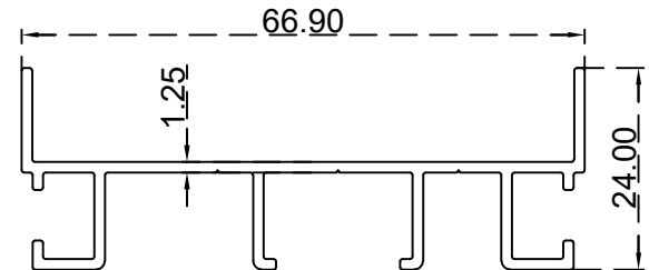
جنب مجريين و نصف عادي بدون يو الرقم التسلسلي للصنف: BLT1569 الوزن ( Kg/m ) : 0.5470
