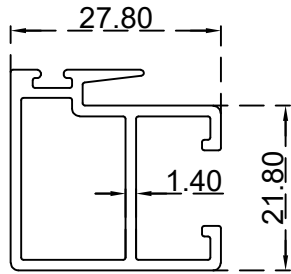
شوليف عادي (6-3) ملم الرقم التسلسلي للصف: ZD019 الوزن (Kg/m): 0.4750
