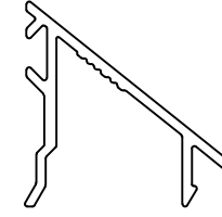
كليبس ماييل زجاج دبل الرقم التسلسلي للصنف: BLT4833 الوزن 0.221:(Kg/m)
