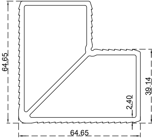
زاوية جمع (66 / 66) 2000 الرقم التسلسلي للصنف: WJM51.8C الوزن (Kg/m): 3.269
