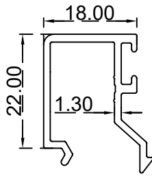
كليبس دربزين مستطيل الرقم التسلسلي للصنف: AS00027 الوزن 0.292:(Kg/m)
