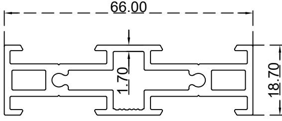
عمود (66-18) ملم الرقم التسلسلي للصنف: BLT409 الوزن 1.040: (Kg/m)
