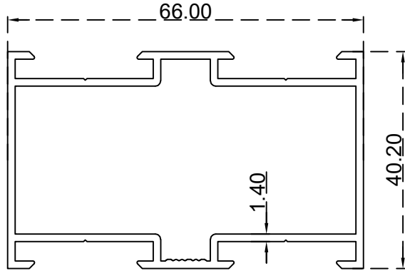
عمود (66-40) ملم الرقم التسلسلي للصنف: BLT047 الوزن 0.954: (Kg/m)
