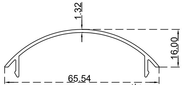
غطاء مدور الرقم التسلسلي للصنف: BLT368 الوزن 0.325: (Kg/m)
