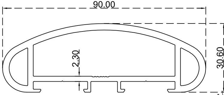
دريزين 90 ملم الرقم التسلسلي للصنف: BLT4377 الوزن 1.761:(Kg/m)
