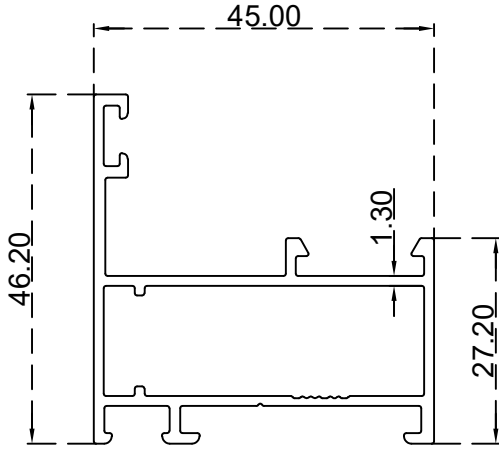
حلق 30 ملم الرقم التسلسلي للصنف: BLT3153 الوزن 0.690:(Kg/m)
