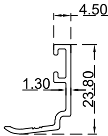
كلبس 4.5 ملم الرقم التسلسلي للصنف: BLT3416 الوزن 0.164:(Kg/m)
