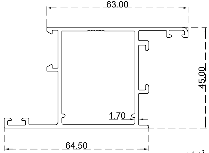
دفة باب الرقم التسلسلي للصنف: BLT3387 الوزن 1.090:(Kg/m)
