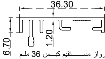
برواز مستقيم كبس 36 ملم الرقم التسلسلي للصنف: BLT4020 الوزن 0.263:(Kg/m)
