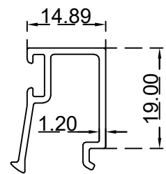
كلبس 15 ملم الرقم التسلسلي للصنف: BLT1587 الوزن 0.232:(Kg/m)
