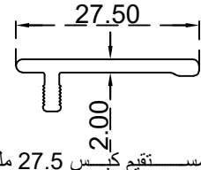
برواز مستقيم كبس 27.5 ملم الرقم التسلسلي للصنف: BLT869 الوزن 0.190:(Kg/m)
