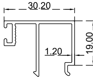
كلبس 30 ملم الرقم التسلسلي للصنف: BLT3353 الوزن 0.315:(Kg/m)
