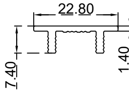
تي دبل الرقم التسلسلي للصنف: BLT031 الوزن 0.158:(Kg/m)
