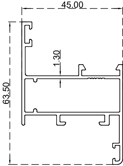
حلق إدفة الرقم التسلسلي للصنف: BLT3348 الوزن 0.797:(Kg/m)
