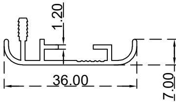
برواز كبس 36 ملم الرقم التسلسلي للصنف: BLT040 الوزن 0.251:(Kg/m)
