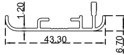
برواز كبس 43 ملم الرقم التسلسلي للصنف: BLT4782 الوزن 0.271:(Kg/m)
