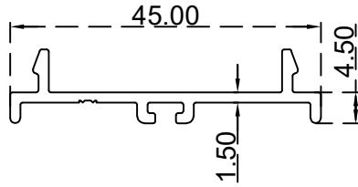
غطاء تحتون باب مع فرشاية الرقم التسلسلي للصنف: BLT3487 الوزن 0.295:(Kg/m)
