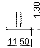
تي تسكيرة الرقم التسلسلي للصنف: BLT3660 الوزن 0.086:(Kg/m)
