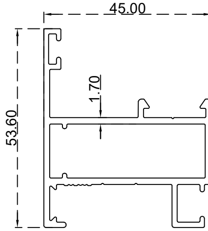
حلق منوبلوك 30 ملم الرقم التسلسلي للصنف: BLT1592A الوزن 0.896:(Kg/m)
