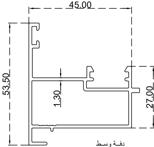
دفة وسط الرقم التسلسلي للصنف: BLT1928 الوزن 0.737:(Kg/m)
