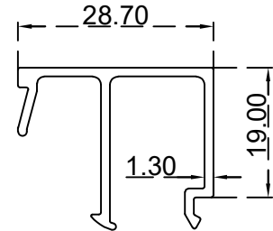
كلبس 29 ملم الرقم التسلسلي للصنف: BLT3418 الوزن 0.314:(Kg/m)
