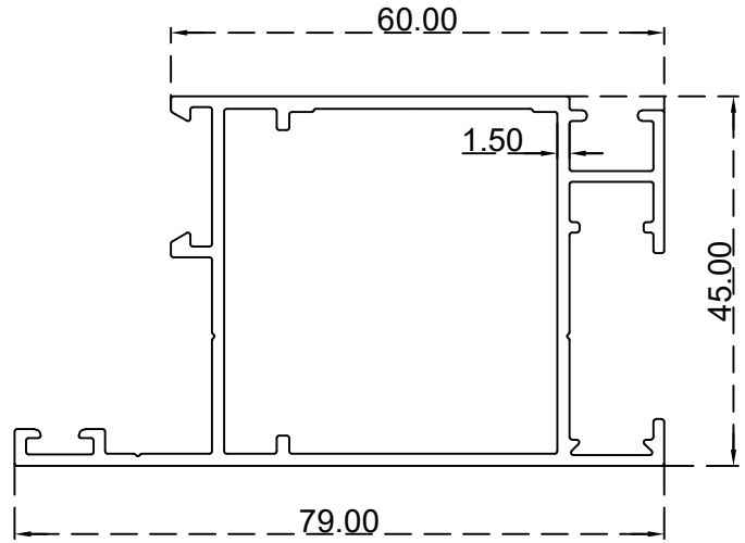
حلق منوبلوك 60 ملم الرقم التسلسلي للصنف: BLT860 الوزن 0.969:(Kg/m)
