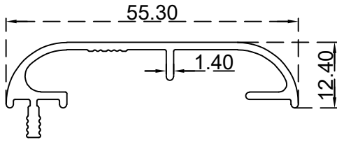
برواز كبس 50 ملم الرقم التسلسلي للصنف: BLT622 الوزن 0.421:(Kg/m)
