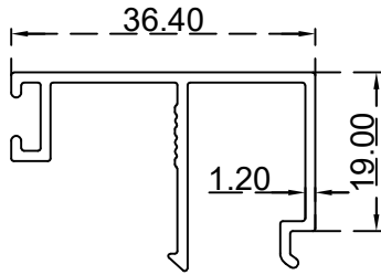
كلبس 36 ملم الرقم التسلسلي للصنف: BLT397 الوزن 0.335:(Kg/m)
