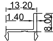
كابس سد ماء الرقم التسلسلي للصنف: BLT3328 الوزن 0.081:(Kg/m)
