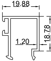
كلبس 20 ملم الرقم التسلسلي للصنف: BLT060A الوزن (Kg/m): 0.245
