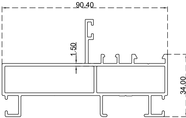
ثابت مجريين 90 ملم الرقم التسلسلي للصنف: BLT3183 الوزن 1.354:(Kg/m)
