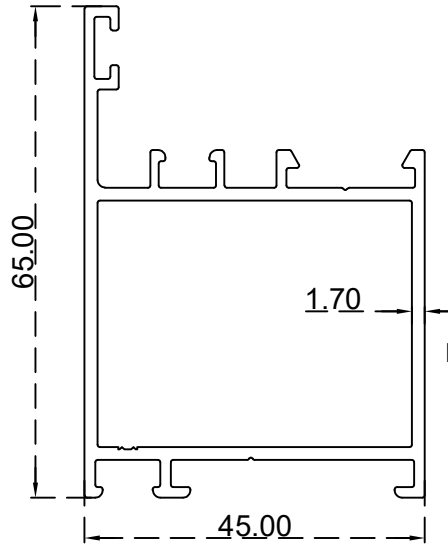
حلق مع بروز 20 ملم الرقم التسلسلي للصنف: BLT394 الوزن 1.053:(Kg/m)
