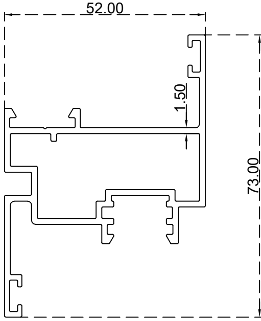
دفة دمج فتحة خارجية الرقم التسلسلي للصنف: BLT2005 الوزن 1.092:(Kg/m)
