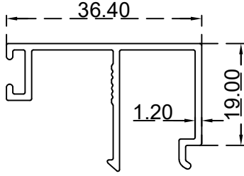
كابس 36 ملم الرقم التسلسلي للصنف: BLT397 الوزن 0.335:(Kg/m)
