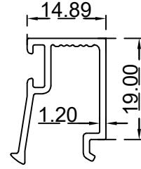
كابس 15 ملم الرقم التسلسلي للصنف: BLT1587 الوزن 0.232:(Kg/m)
