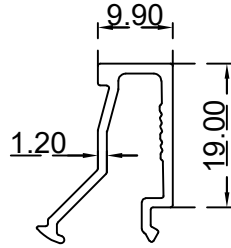
كلبس 10 ملم الرقم التسلسلي للصنف: BLT3368 الوزن (Kg/m): 0.225
