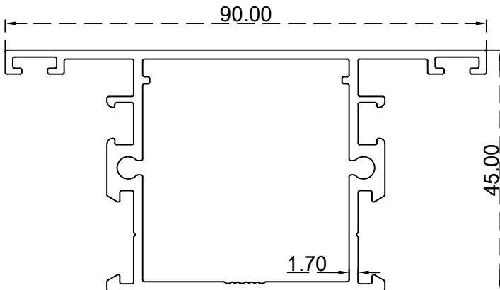
قاطع برغي 90ملم الرقم التسلسلي للصنف: BLT1595 الوزن 1.309:(Kg/m)
