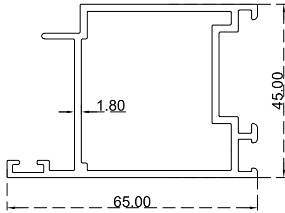
حلق باب منوبلوك الرقم التسلسلي للصنف: BLT3426 الوزن 1.104:(Kg/m)
