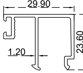
كابس 30 ملم الرقم التسلسلي للصنف: BLT3353 الوزن 0.325:(Kg/m)
