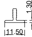
تي تسكيرة الرقم التسلسلي للصنف: BLT3660 الوزن (Kg/m): 0.086
