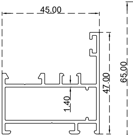
حلق 30 ملم الرقم التسلسلي للصنف: BLT352 الوزن 0.763:(Kg/m)
