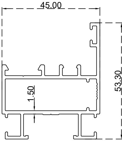
حلق منوبلوك 35 ملم الرقم التسلسلي للصنف: BLT392 الوزن 0.891:(Kg/m)
