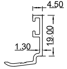
كليس 4.5 ملم الرقم التسلسلي للصنف: BLT3416 الوزن 0.164:(Kg/m)
