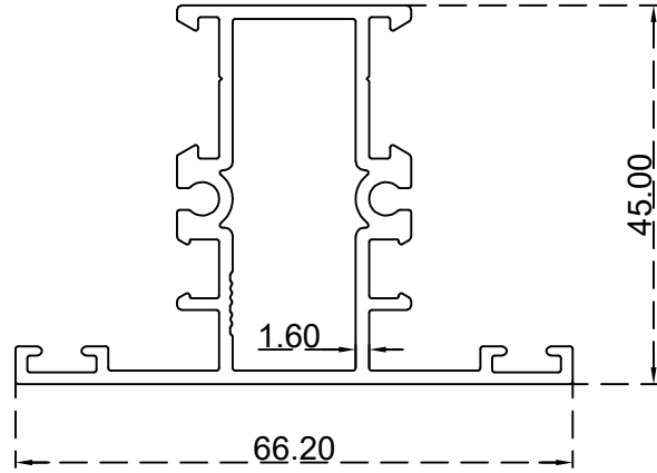
قاطع مع برغي 66 ملم الرقم التسلسلي للصنف: BLT395B الوزن 1.083:(Kg/m)
