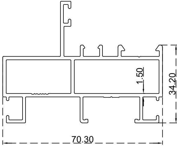
ثابت مجريين 70 ملم الرقم التسلسلي للصنف: BLT377 الوزن 1.182:(Kg/m)
