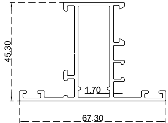
حلق فتحة خارجية الرقم التسلسلي للصنف: BLT1651 الوزن 1.009:(Kg/m)
