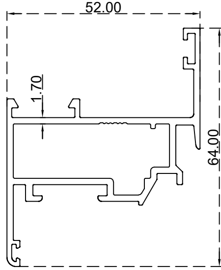
دفة الرقم التسلسلي للصنف: BLT353B الوزن 1.014:(Kg/m)
