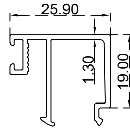
كلبس 26 ملم الرقم التسلسلي للصنف: BLT059B الوزن (Kg/m): 0.312
