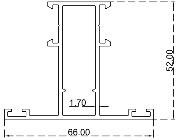
قاطع دفة 66ملم الرقم التسلسلي للصنف: BLT1929 الوزن 0.989:(Kg/m)
