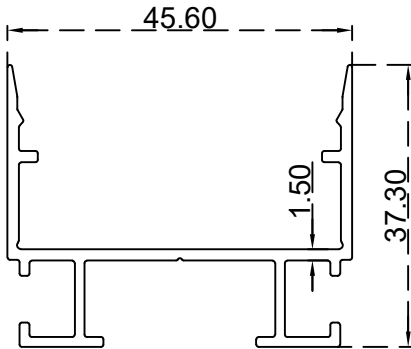
تحويلة حلق الرقم التسلسلي للصنف: BLT3185 الوزن 0.569:(Kg/m)
