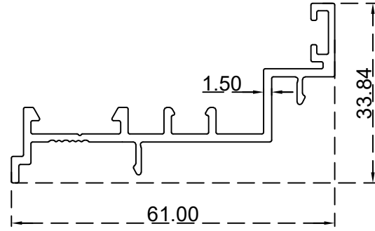
تحويل دفة لشباك الرقم التسلسلي للصنف: BLT4639 الوزن 0.531:(Kg/m)
