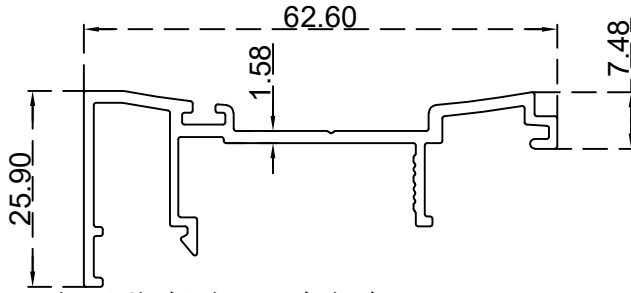
تحويل حلق فتحة داخلية/خارجية الرقم التسلسلي للصنف: BLT3595 الوزن 0.541:(Kg/m)
