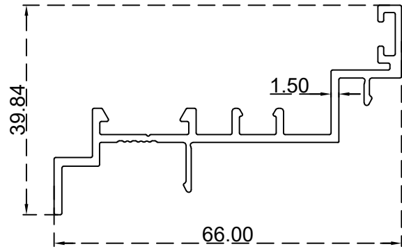
تحويل حلق لشباك الرقم التسلسلي للصنف: BLT4640 الوزن 0.590:(Kg/m)
