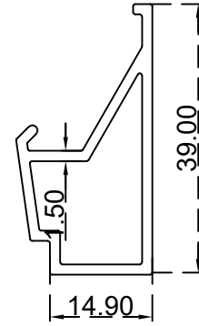
كابس حلق زجاج (16-11) ملم الرقم التسلسلي للصنف: BLT1982 الوزن 0.419:(Kg/m)
