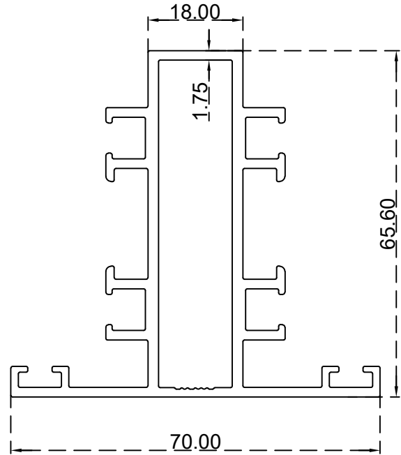
قاطع حلق رفيع الرقم التسلسلي للصنف: BLT1974 الوزن 1.606:(Kg/m)
