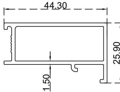
كابس حلق زجاج (11-6) ملم الرقم التسلسلي للصنف: BLT1960 الوزن 0.548:(Kg/m)
