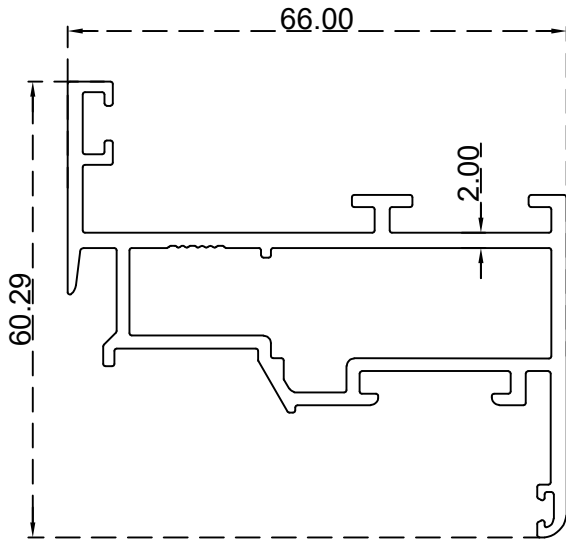
دفة الرقم التسلسلي للصنف: BLT4641 الوزن 1.278:(Kg/m)
