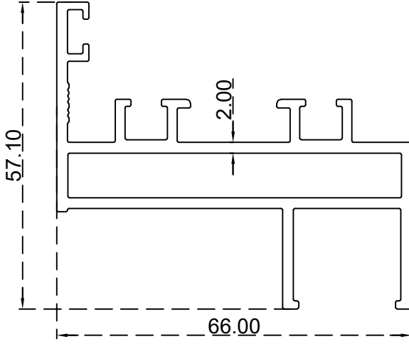
حلق واجهة زجاجية الرقم التسلسلي للصنف: BLT4501 الوزن 1.425:(Kg/m)
