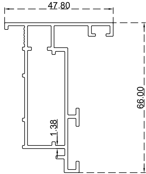
تحويل دفة الرقم التسلسلي للصنف: BLT3557 الوزن 0.896:(Kg/m)
