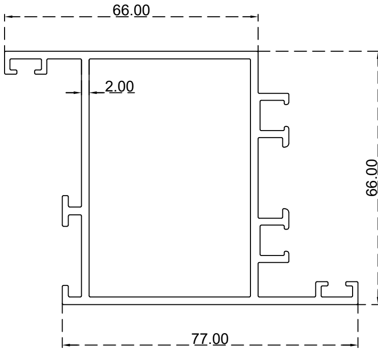
حلق إدفة الرقم التسلسلي للصنف: BLT1971 الوزن 1.814:(Kg/m)
