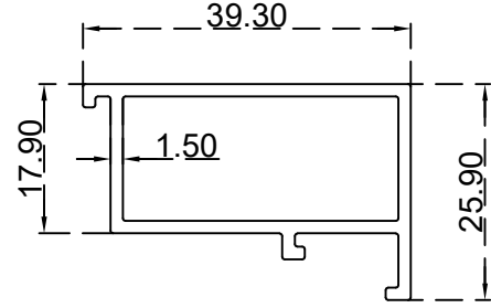
كابس حلق زجاج (16-11) ملم الرقم التسلسلي للصنف: BLT1963 الوزن 0.490:(Kg/m)
