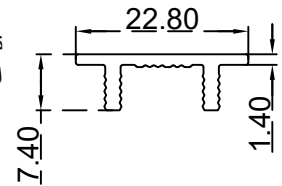
تي دبل الرقم التسلسلي للصنف: BLT031 الوزن 0.158:(Kg/m)
