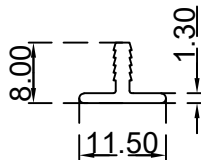
تي تسكيرة الرقم التسلسلي للصنف: BLT3660 الوزن 0.086:(Kg/m)
