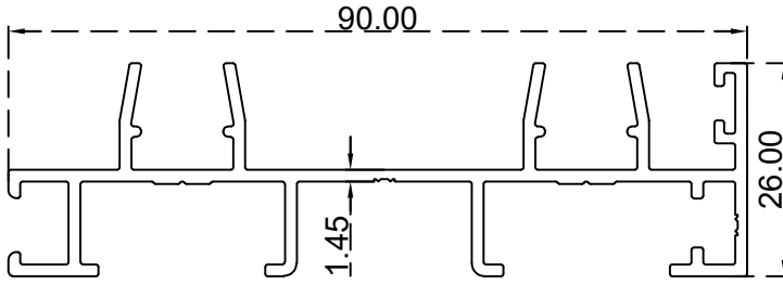
مجرى واحد داخلي بانوراما الرقم التسلسلي للصنف: BLT613 الوزن 1.057:(Kg/m)
