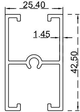
قاطع طولي 8 ملم الرقم التسلسلي للصنف: BLT381 الوزن 0.556:(Kg/m)
