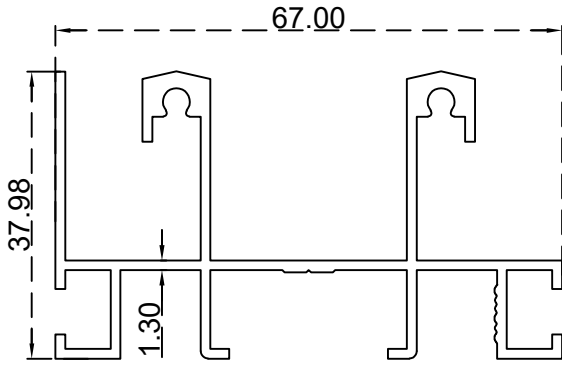
عليون مجريين مفتوح الرقم التسلسلي للصنف: BLT002 الوزن (Kg/m): 0.965
