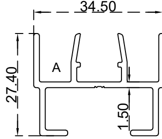
جانب مجرى واحد 35 ملم الرقم التسلسلي للصنف: BLT3321 الوزن 0.506:(Kg/m)
