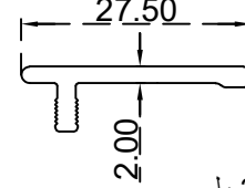
برواز مسـتقيم 27.5 ملم الرقم التسلسلي للصف: BLT869 الوزن 0.190:(Kg/m)
