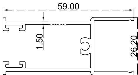
تحتون زجاج 18 ملم الرقم التسلسلي للصف: BLT3330 الوزن 0.713:(Kg/m)
