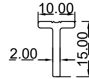
تي مقوي امباطيا الرقم التسلسلي للصنف: BLT3511 الوزن 0.119:(Kg/m)
