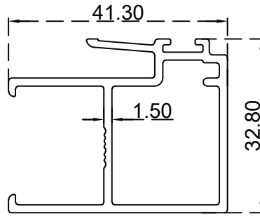
شوليف دبل 14 ملم الرقم التسلسلي للصف: BLT3356 الوزن 0.654:(Kg/m)
