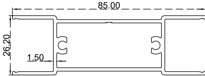
قاطع عرضي دبل زجاج 18 ملم الرقم التسلسلي للصف: BLT3333 الوزن 0.986:(Kg/m)
