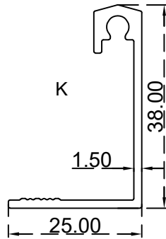
ارضية مجرى واحد 38 ملم الرقم التسلسلي للصف: BLT3508 الوزن 0.342:(Kg/m)
