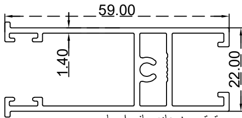
تحتون عادي بانوراما الرقم التسلسلي للصنف: BLT357 الوزن 0.735:(Kg/m)
