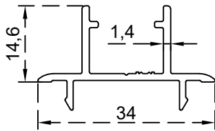
نوشيك اربع دفات الرقم التسلسلي للصنف: BLT1758 الوزن 0.265: (Kg/m)
