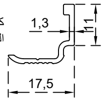
كليبس دفعة زجاج (33-28) ملم الرقم التسلسلي للصنف: BLT3600 الوزن (Kg/m): 0.115
