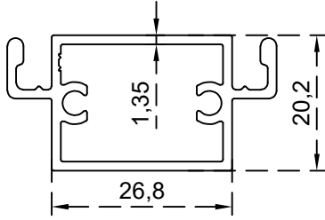
قاطع منخل الرقم التسلسلي للصنف: BLT1757 الوزن 0.517: (Kg/m)
