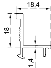
كليبس ثابت زجاج (18-13) ملم الرقم التسلسلي للصنف: BLT3163 الوزن (Kg/m): 0.190
