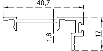
شوليف منخل الرقم التسلسلي للصنف: BLT1780 الوزن 0.310: (Kg/m)
