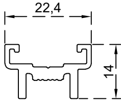
مجرى فلاح الرقم التسلسلي للصنف: BLT1770 الوزن 0.273: (Kg/m)
