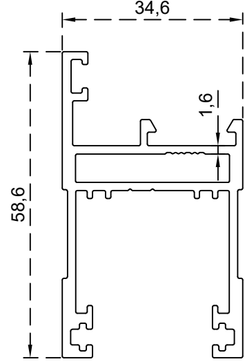
دفة الرقم التسلسلي للصنف: BLT1777 الوزن 0.992: (Kg/m)
