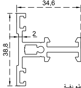
قاطع دفة الرقم التسلسلي للصنف: BLT1754 الوزن 0.655: (Kg/m)
