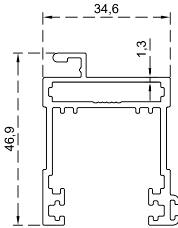
دفة منخل مع فرشاية الرقم التسلسلي للصنف: BLT1885 الوزن 0.845: (Kg/m)
