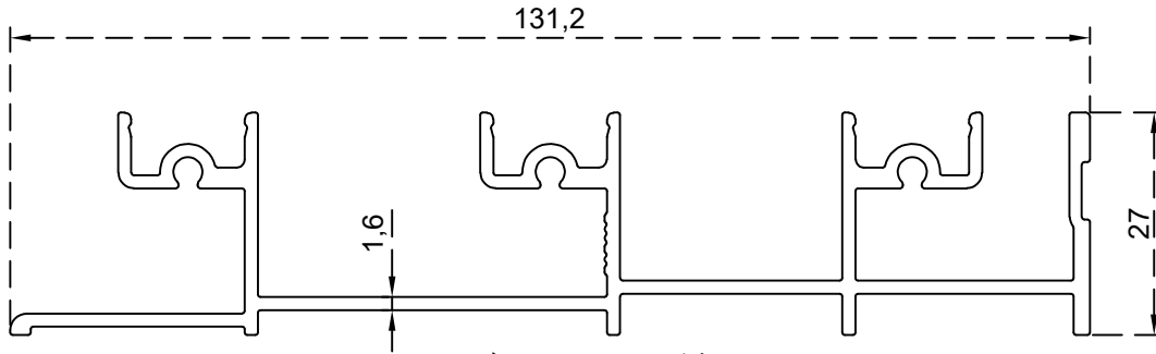
ارضية ثلاث مجاري 27 ملم الرقم التسلسلي للصنف: BLT1762 الوزن (Kg/m): 1.445
