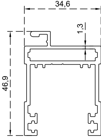
دفة منخل الرقم التسلسلي للصنف: BLT1779 الوزن 0.826: (Kg/m)
