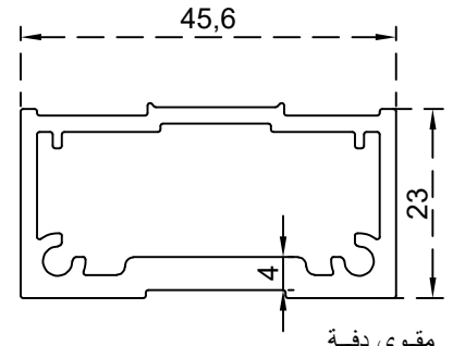
مقوي دفة الرقم التسلسلي للصنف: BLT1755 الوزن 0.963: (Kg/m)
