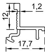
كليبس دفعة زجاج (11-7) ملم الرقم التسلسلي للصنف: BLT3567 الوزن (Kg/m): 0.142
