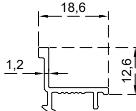
كليبس دفعة زجاج (6-4) ملم الرقم التسلسلي للصنف: BLT3218 الوزن (Kg/m): 0.145
