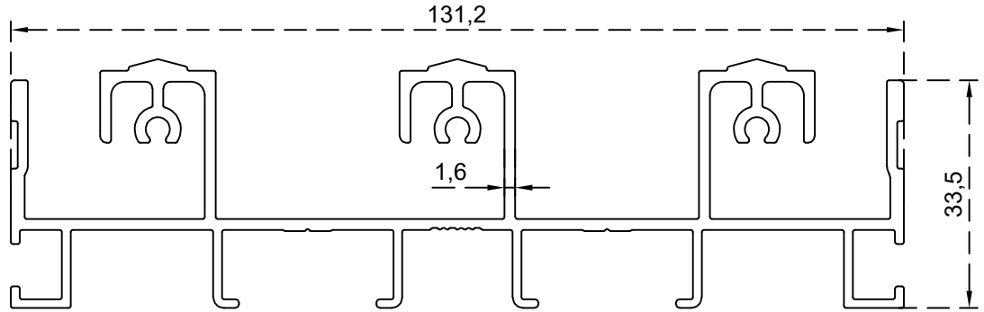
عليون ثلاث مجاري الرقم التسلسلي للصنف: BLT3649 الوزن (Kg/m): 2.057
