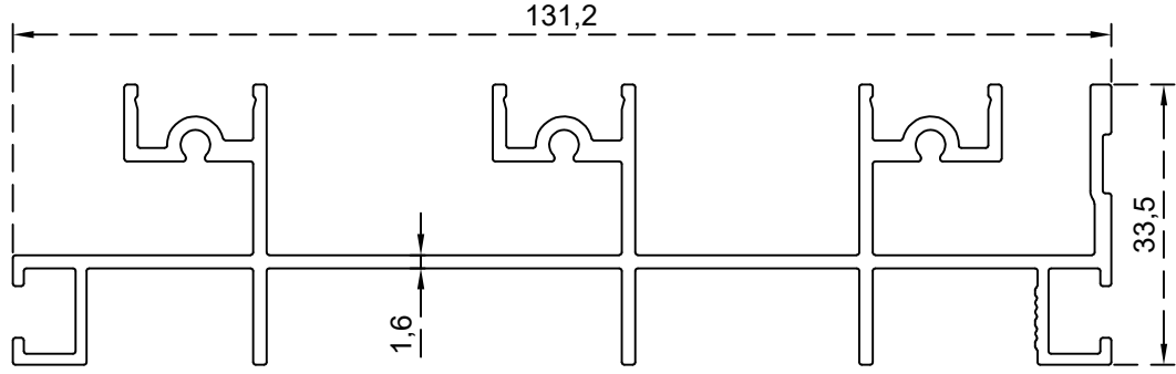
عليون ثلاث مجاري مفتوح الرقم التسلسلي للصنف: BLT3201 الوزن (Kg/m): 1.667
