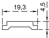
فلاخ الرقم التسلسلي للصنف: BLT1756 الوزن (Kg/m): 0.157
