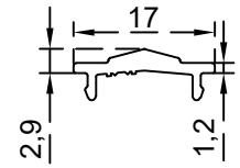
غطاء مجرى الرقم التسلسلي للصنف: BLT1769 الوزن 0.10: (Kg/m)
